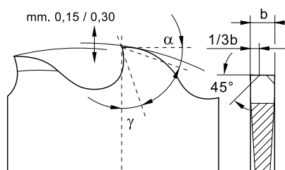
Denti Alternati (BW) su passi 3-4-5 Variable Teeth on 3-4-5 pitch Dents alternées (BW) pour pas 3-4-5
